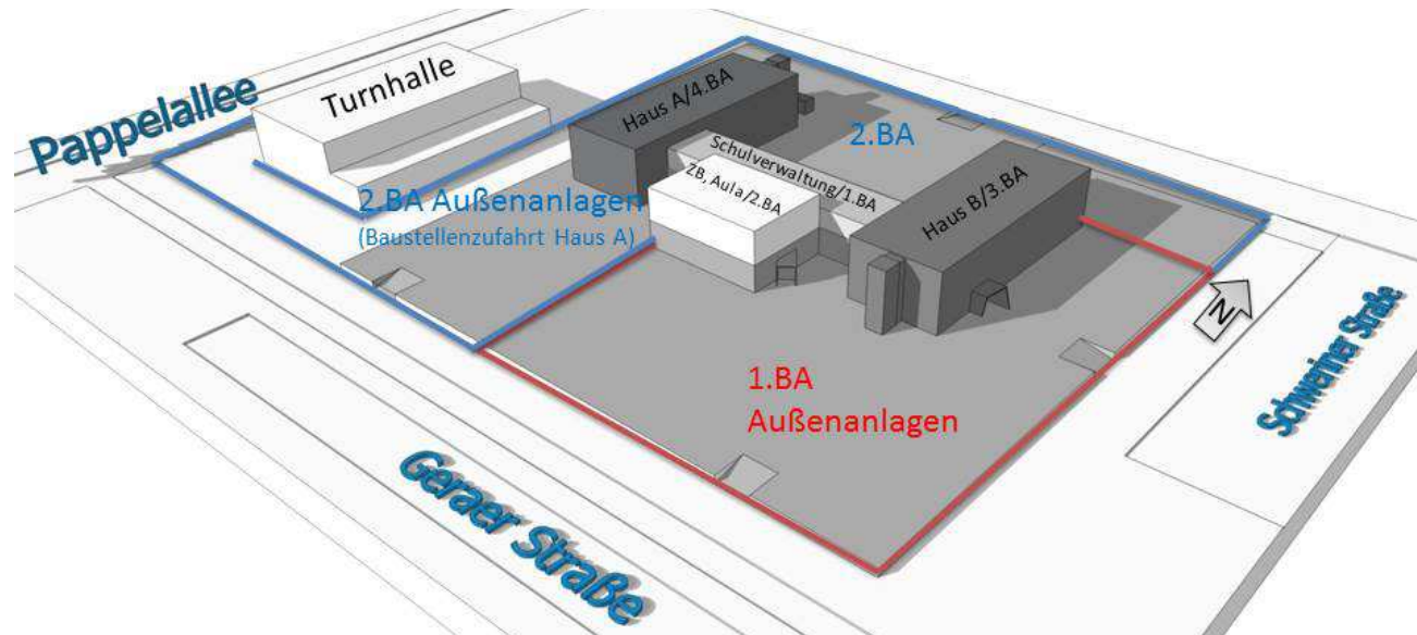
Übersichtsplan Gesamtmaßnahme
