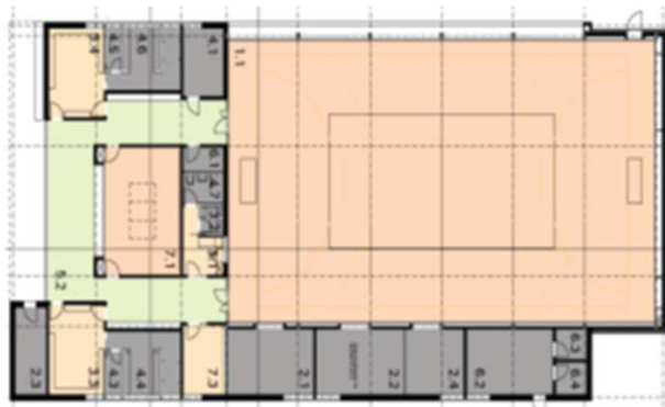
Grundriss Erdgeschoss
