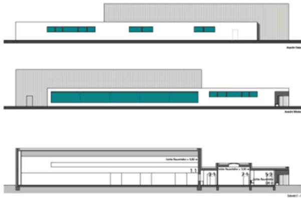
Ansichten, Schnitt
